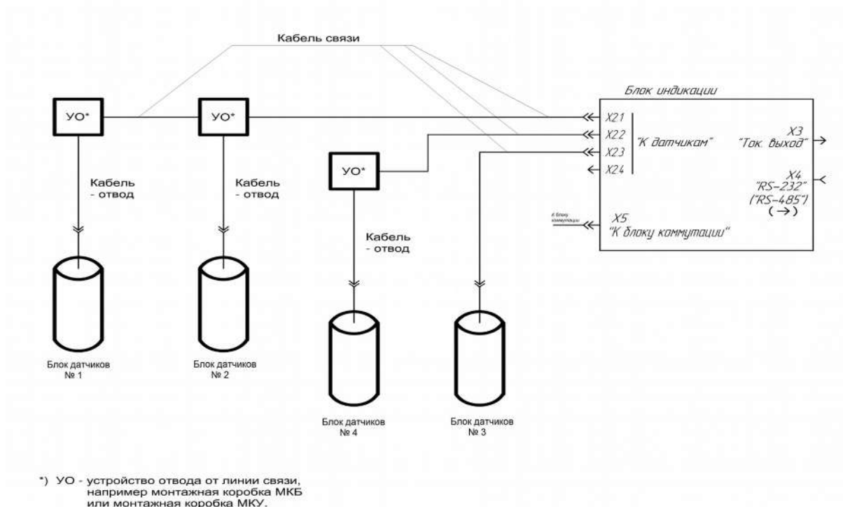
Рис Д.2 Пример смешанного соединения.
